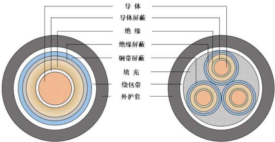
图：电缆产品结构图
