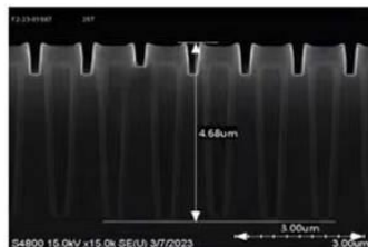
更新一代自对准结构
