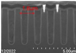
第三代1.6um pitch 结构
