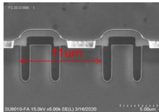
第一代IGBT结构
