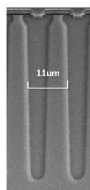
第二代 超级结结构
