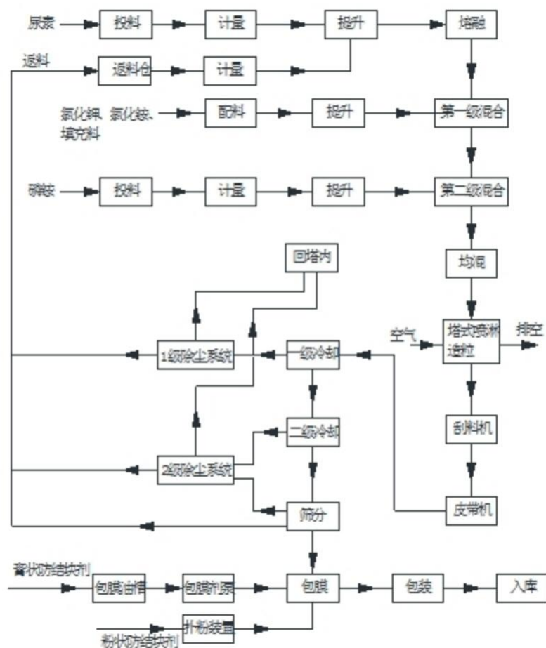
2、磷酸一铵的工艺流程图
