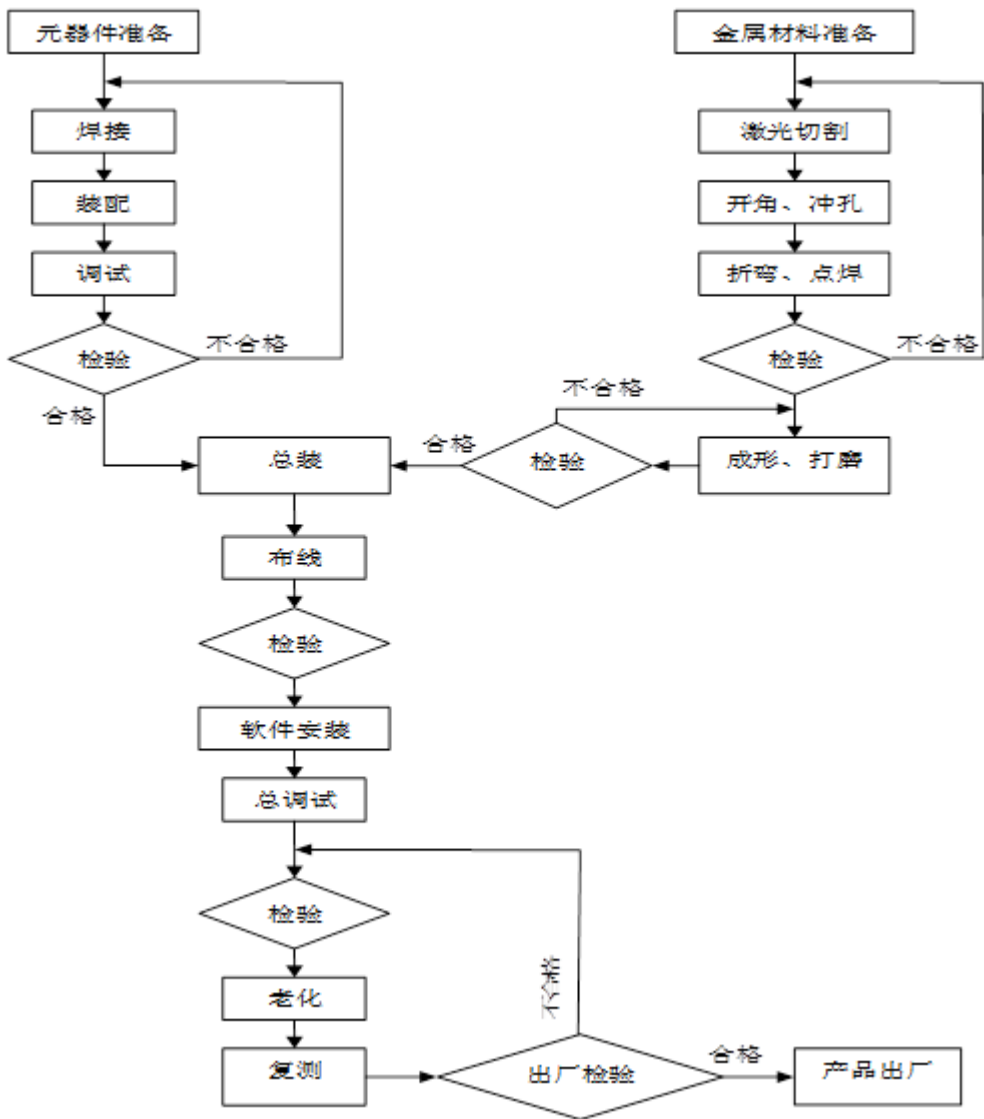
生产流程图
