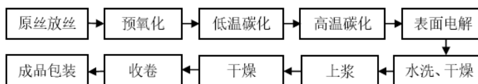
碳纤维制备流程
