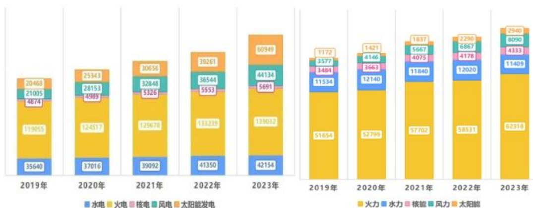
2019年—2023年各类电源累计装机情况 (万千瓦) 2019—2023年规模以上各类电源发电量情况 (亿千瓦时)
