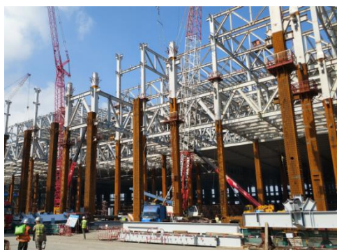
图5：NCC钢结构应用于大型工业厂房
