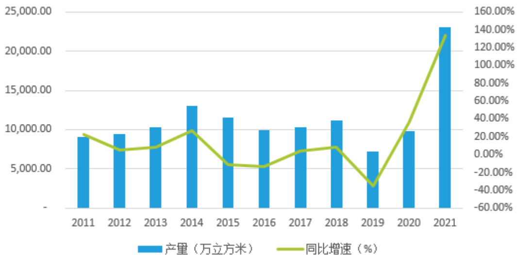
图 9：2011-2021 年全国金属集装箱产量及增长情况
