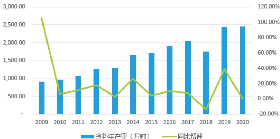
图 8：2009-2020 年我国涂料产量及增长情况
