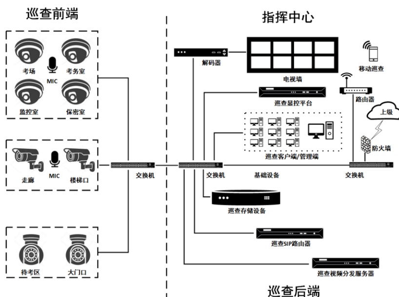
视频监控巡查系统示意图
