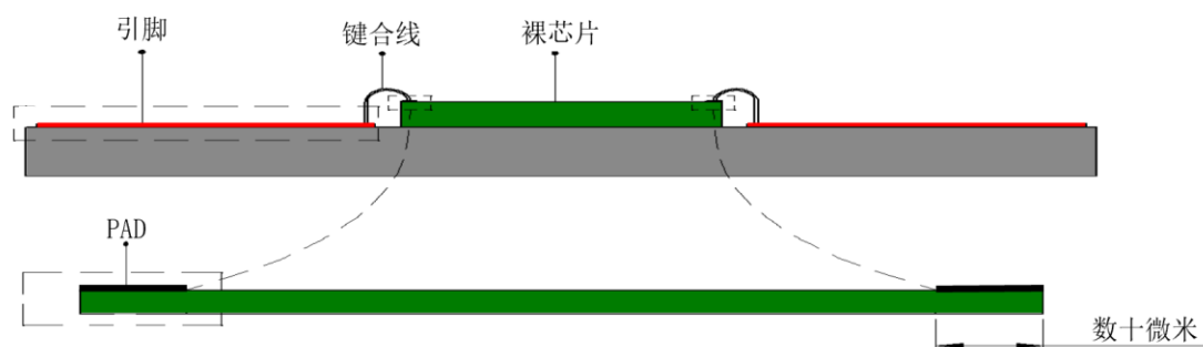
成品芯片及裸芯片截面示意图
