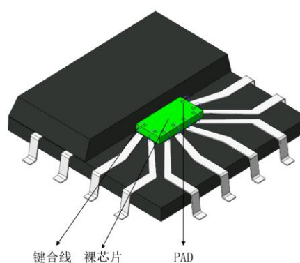
成品芯片局部剖视图（含裸芯片）
