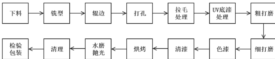
(3) 实木贴皮门板（内门墙板）生产工艺流程
