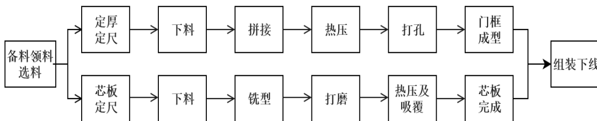
(4) 移门（内门墙板、智能产品）生产工艺流程
