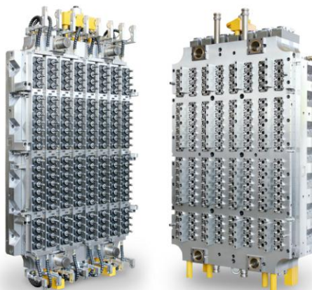
图222-1 176腔瓶坯模具
