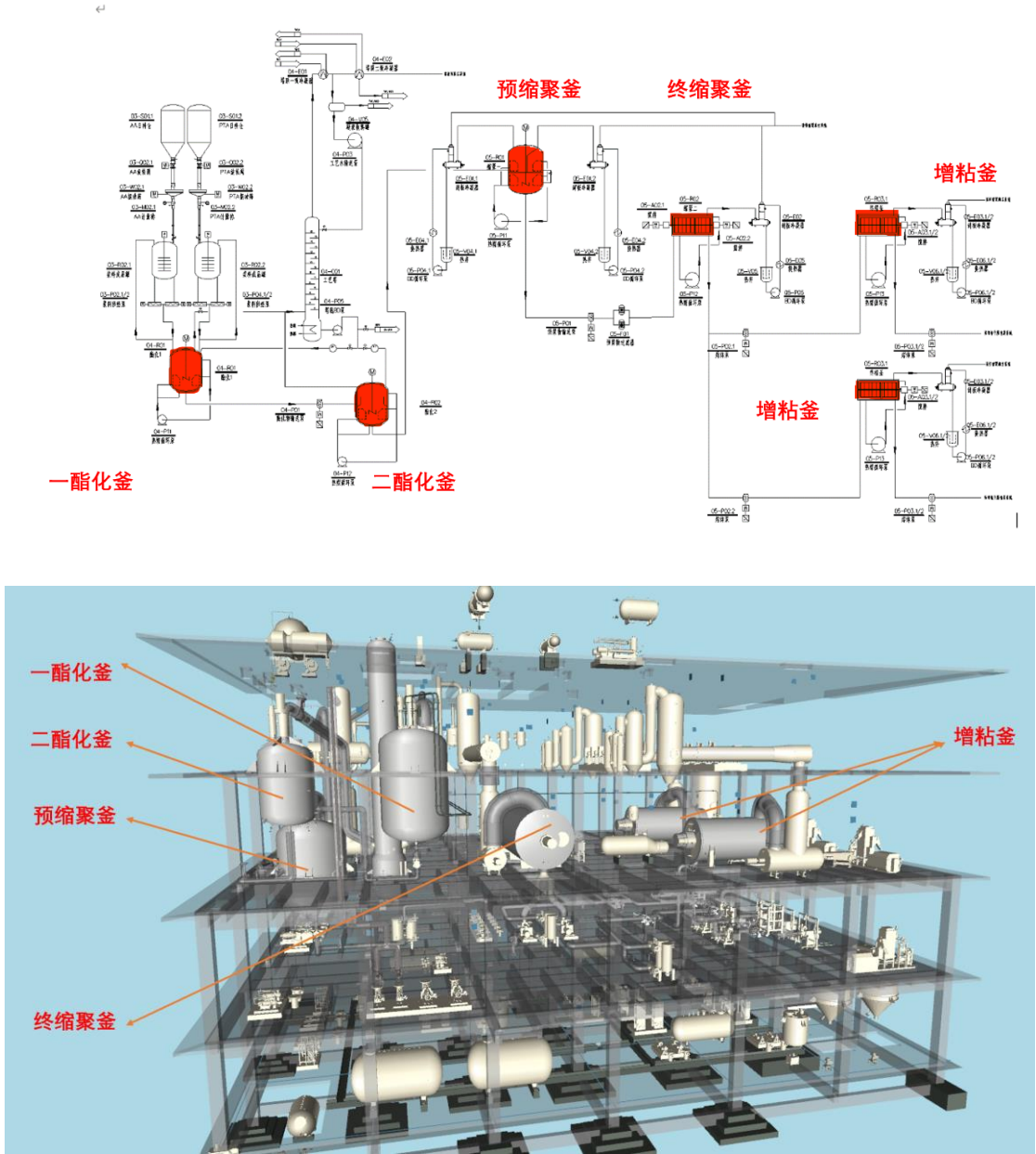
工艺流程图（单线 6 万吨 PBAT 工艺流程示意图）
