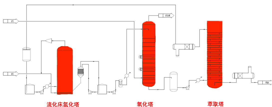
双氧水流化床工艺流程简图
