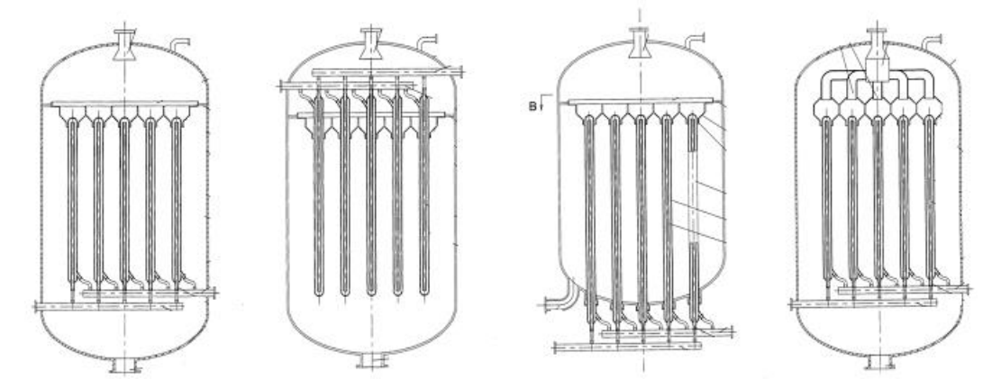
“管状薄膜蒸发器”四种结构示意图
