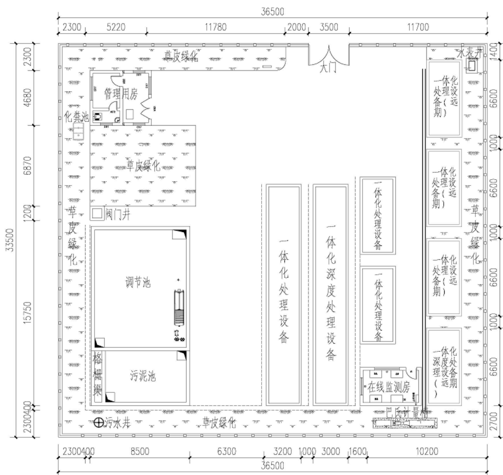
泥窝潭镇污水处理厂平面布置图
