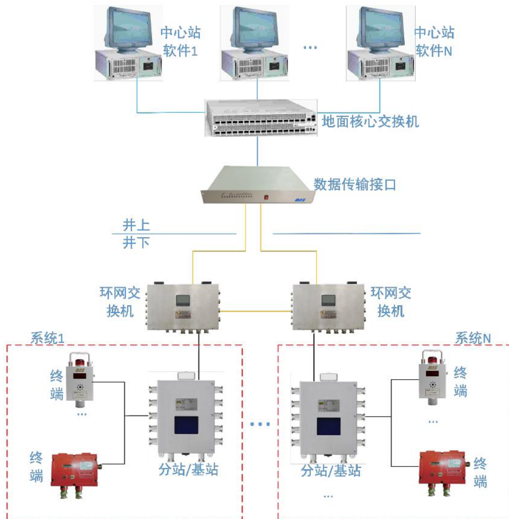
图2-以太网+总线型网络架构
