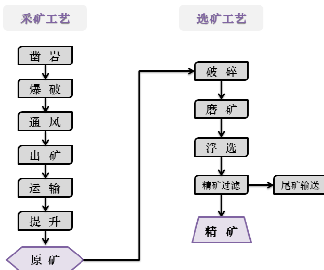
凡口铅锌矿采选工艺流程图
