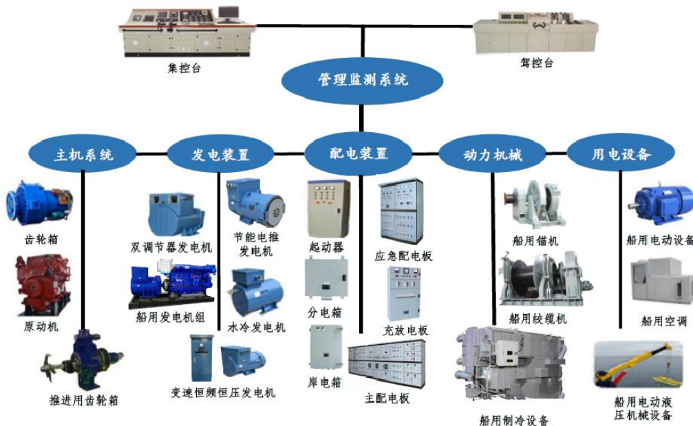
图：船电集成系统硬件设备框架
