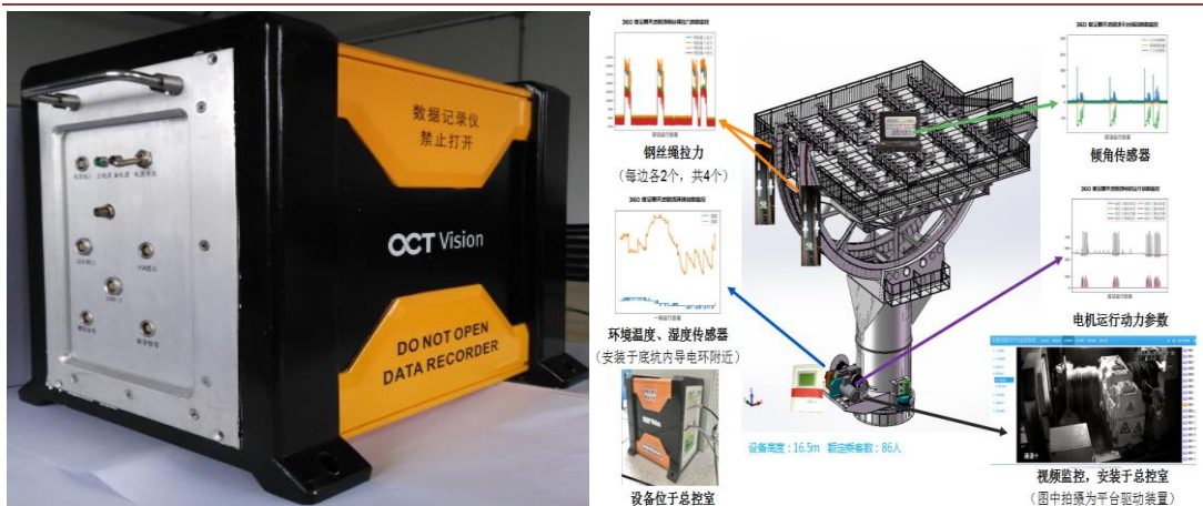
图：“黑匣子”及园区设备性能与监测系统运行示意图
