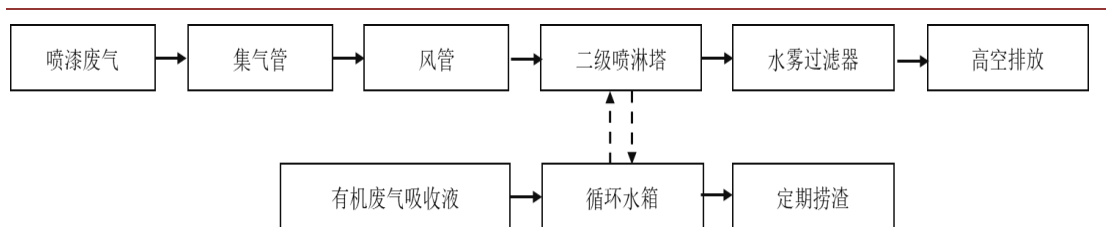
图：废气处理装置工作原理
