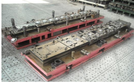
方向盘气囊支架连续模
