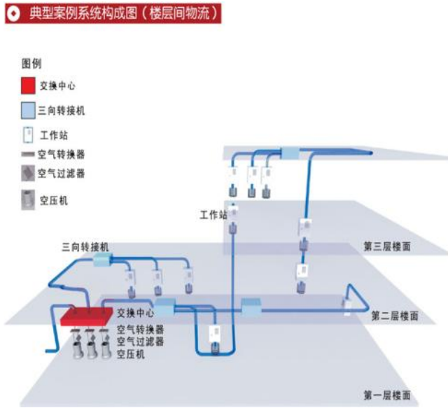
医院气动传输系统
