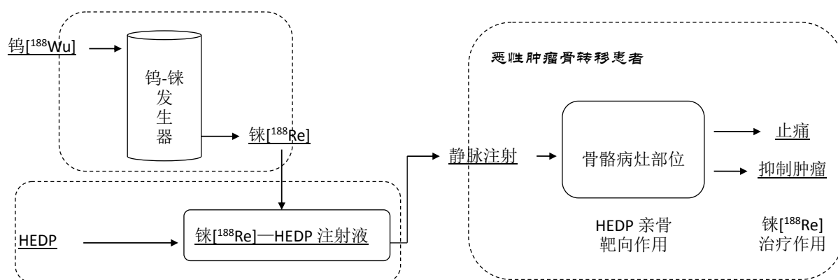
铼 [188Re] -HEDP 注射液临床治疗原理
