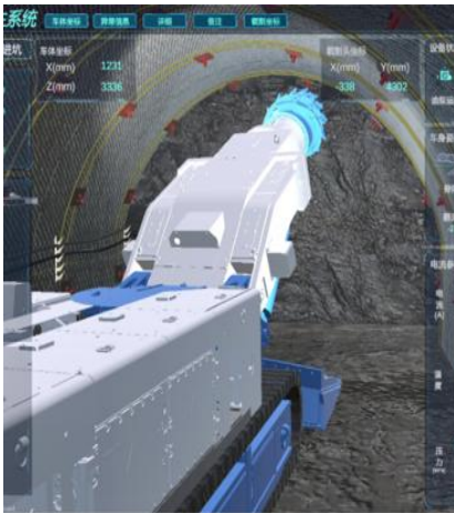
会泽矿业悬臂式掘进机地表远程操控
