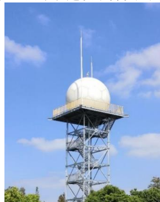
X 波段相控阵天气雷达
