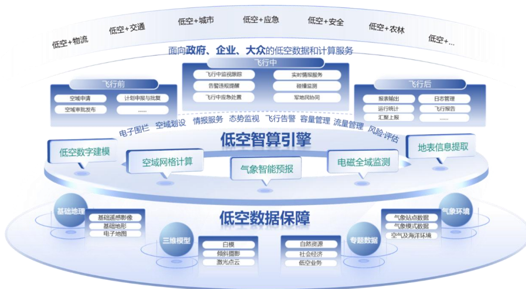
图 3-2 数智低空大脑产品总体架构
