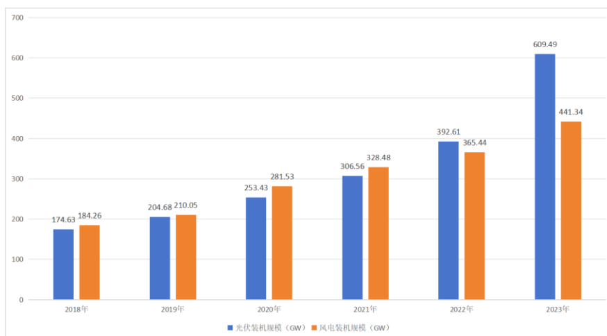
我国 2018-2023 年风电光伏累计装机规模
