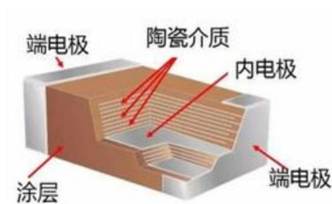
片式多层陶瓷电容器构造
