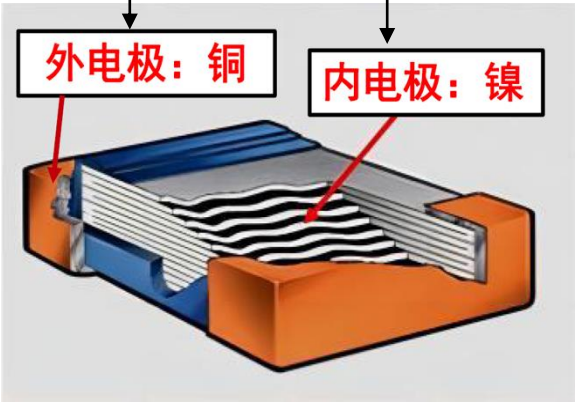
MLCC 剖面图
