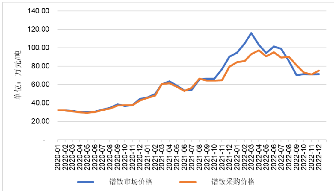
图 5-22 镨钕市场价格与采购价格走势
