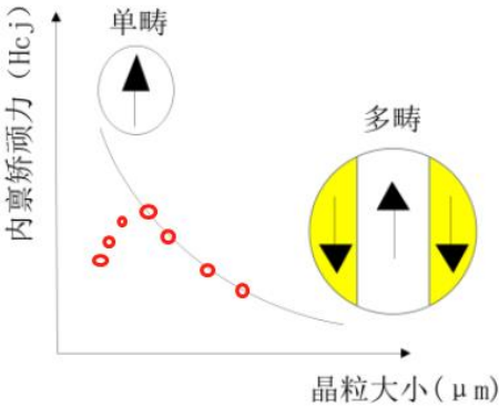
图 5-28 晶粒粒度与矫顽力的关系
