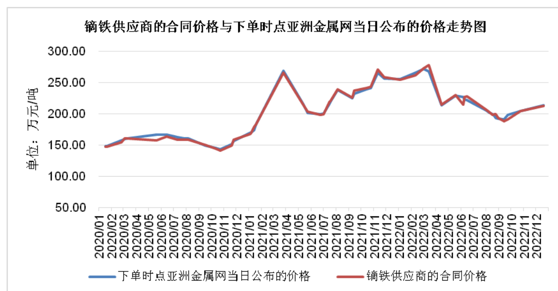
图 5-27 镕铁供应商合同价格与下单时点亚洲金属网当日公布价格走势
