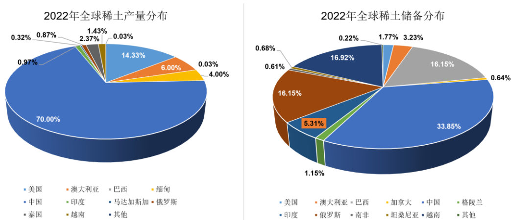
图5-12 全球稀土产量与储备量分布
