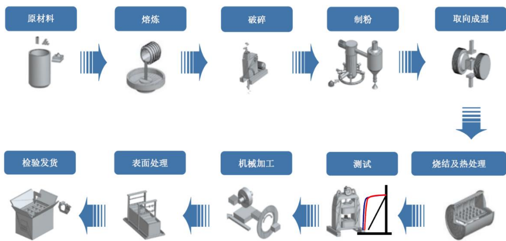
图 5-6 公司烧结钕钴生产工艺流程
