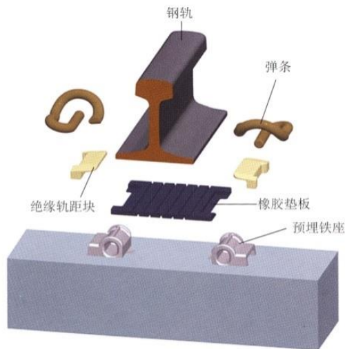
弹条Ⅳ型扣件组装零件图
