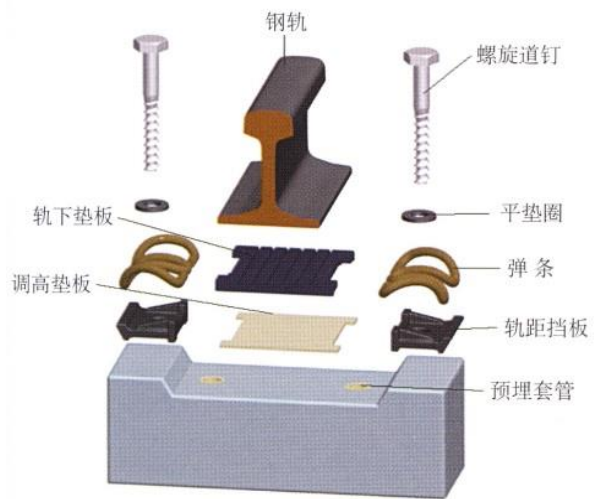
弹条Ⅴ型扣件组装零件图
