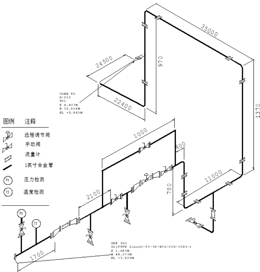
图 2：单线图示例
