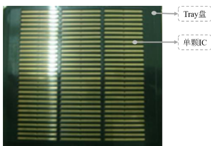
COG 工艺封装出货产品
