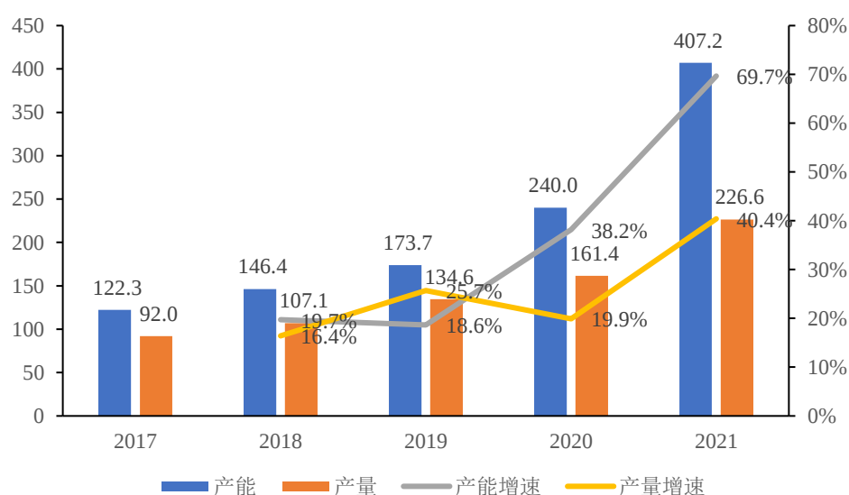
2017-2021 年我国硅片产能/产量及增速（单位：GW）
