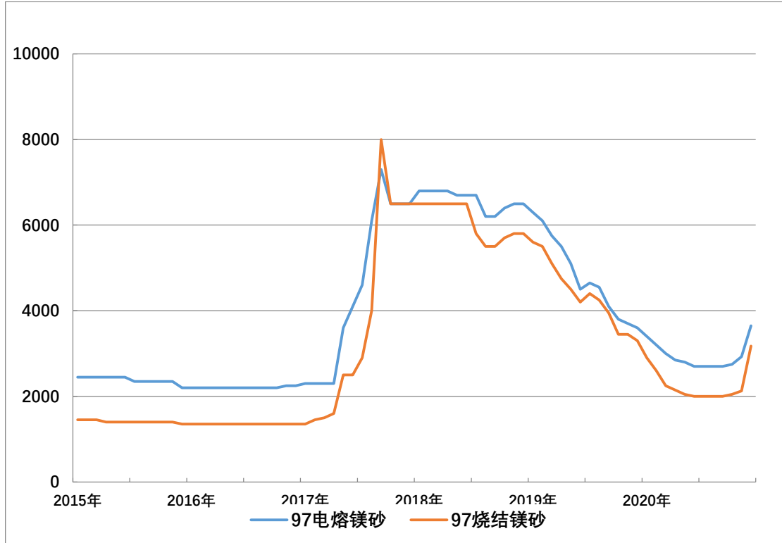
图：2015年-2020年镁砂价格走势
