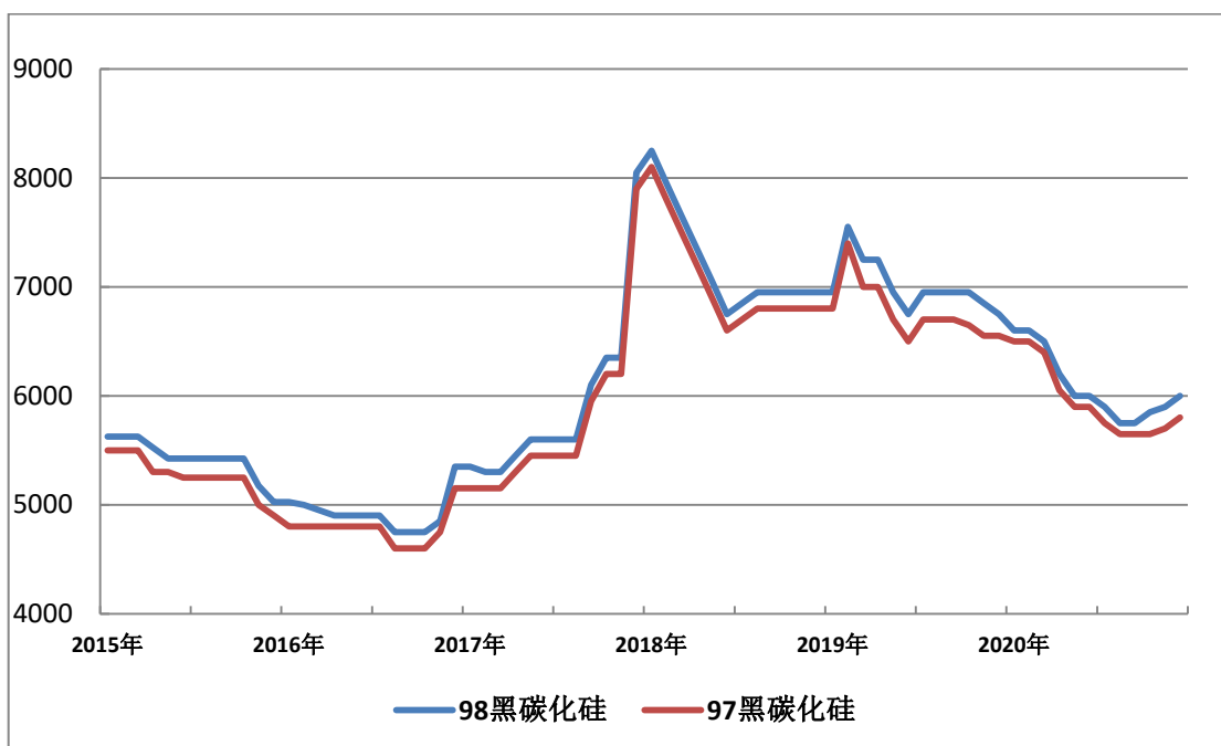
图 2015—2020 年黑碳化硅价格走势图(单位:元/吨)
