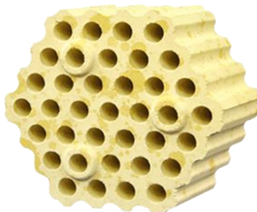
热风炉格子(硅)砖
