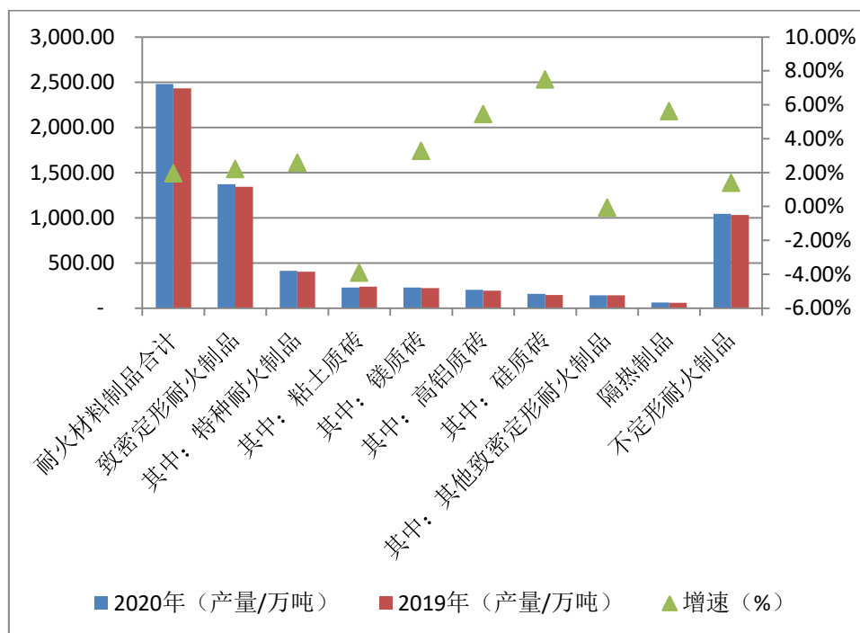
图：2020 年我国耐火材料主要品种产量情况
