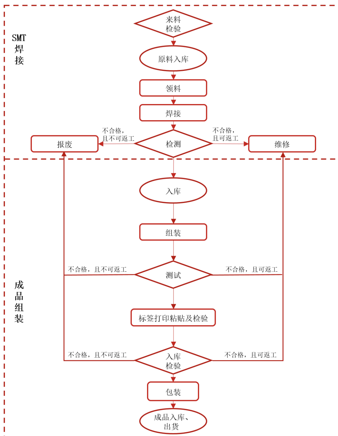
图：电子产品业务工艺流程
