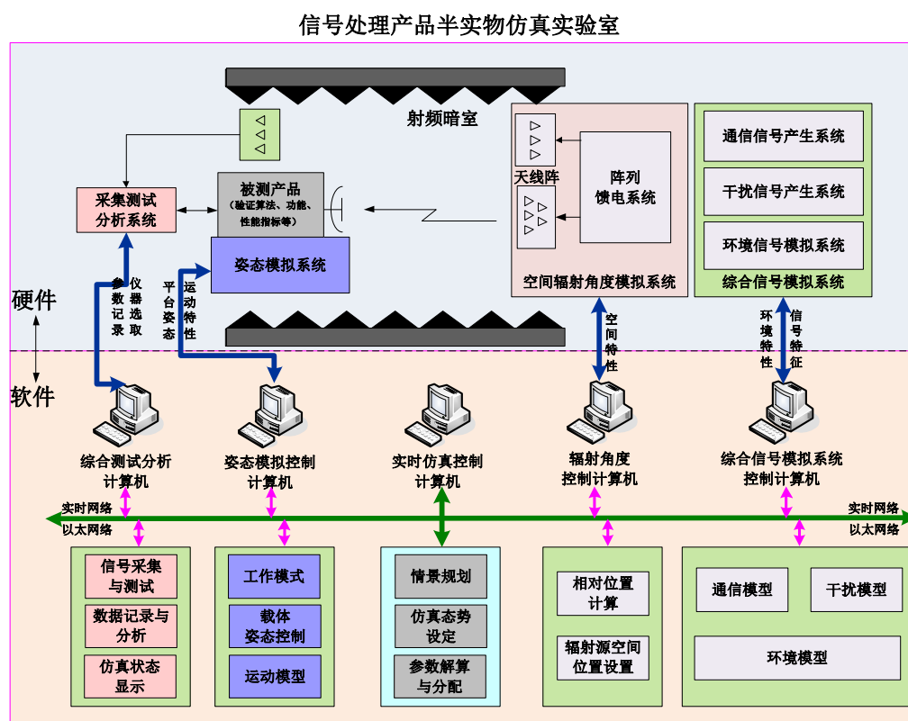
图：发行人信号处理产品仿真验证方案示例
