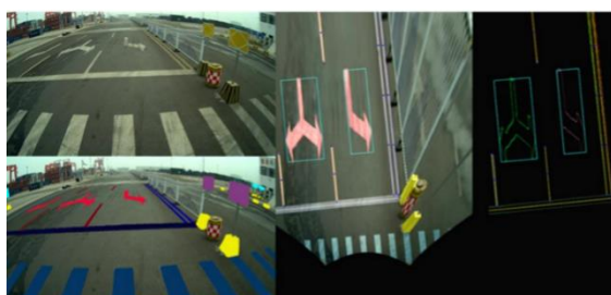
路面标线识别和分割
