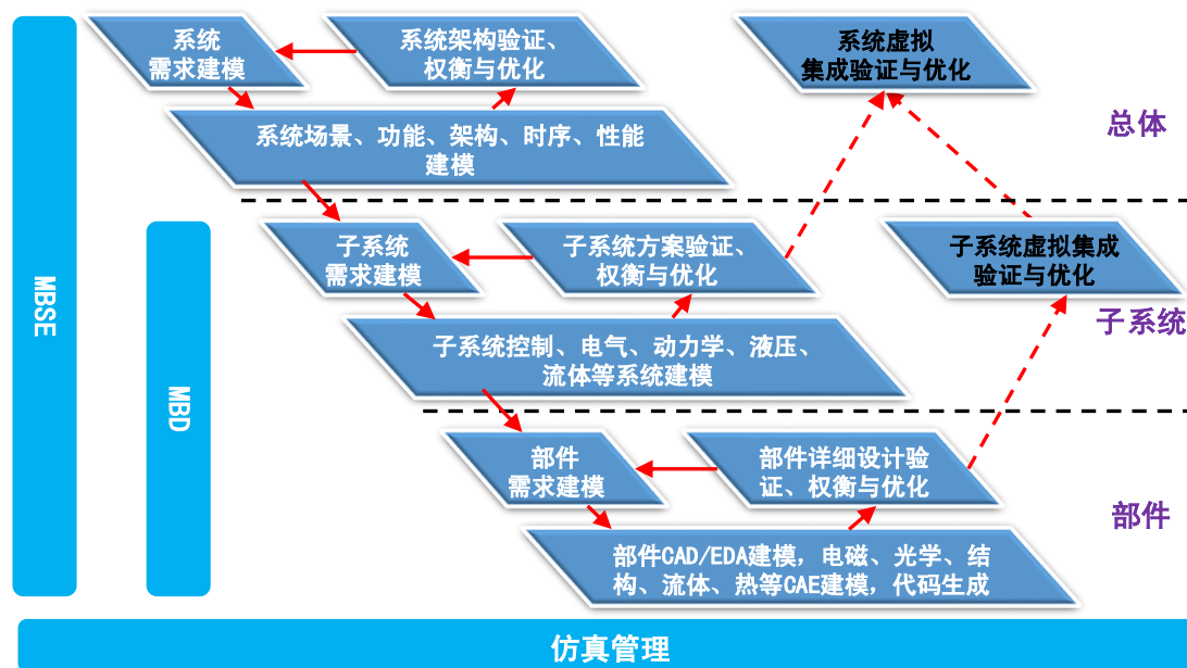
图：发行人多学科建模仿真服务业务
