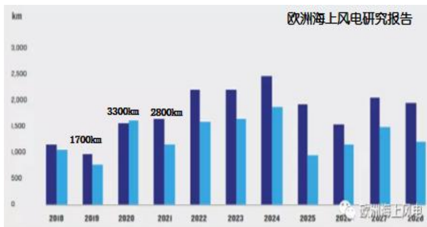
图 4: 2018 年-2028 年全球海上风电海缆安装量 (深蓝色代表中压, 浅蓝色代表高压)
