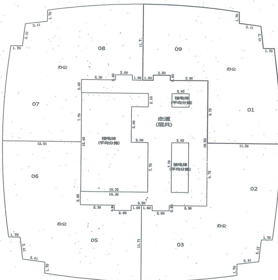
二十六至三十五层平面图
