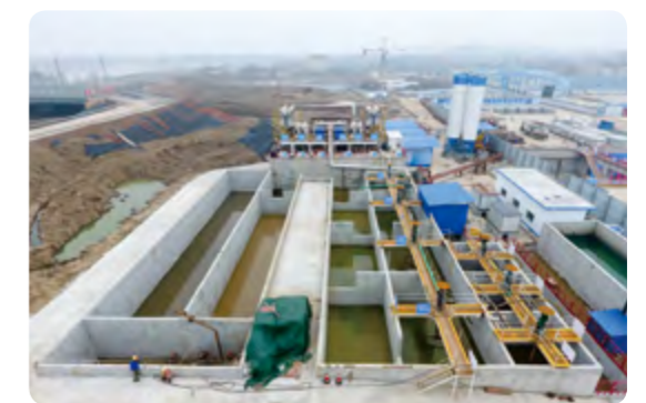
衡阳东洲湘江大桥项目隧道泥水处理场
