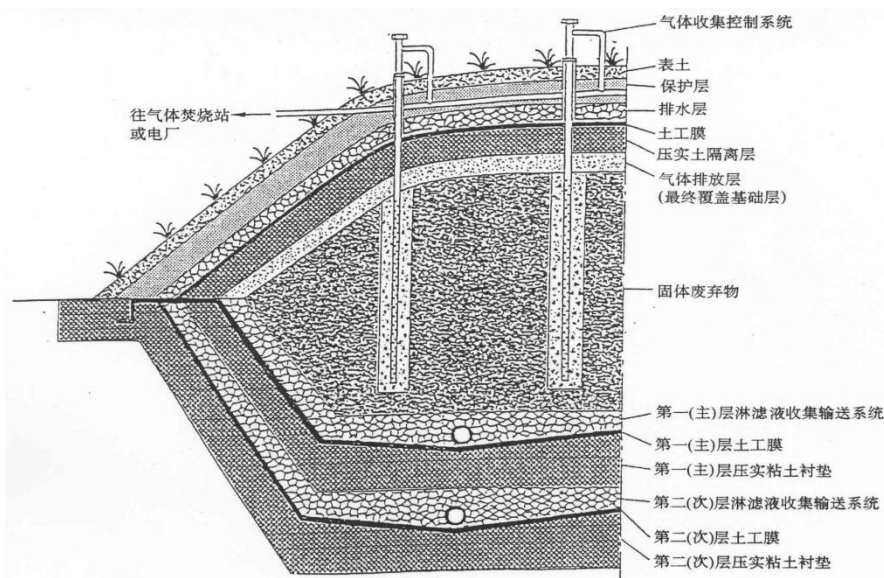
图 1.1 现代卫生填埋场简图
