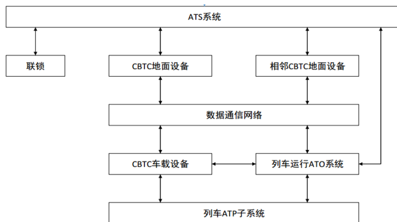
CBTC 结构框图
