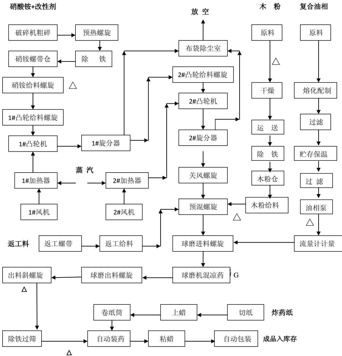
改性铵油炸药连续化自动化生产线工艺流程图
