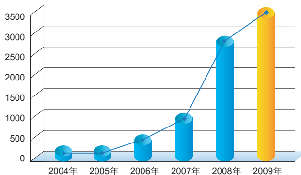
水电机组装机容量（单位：兆瓦）
