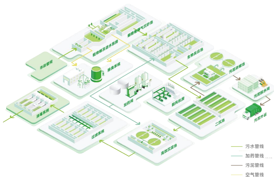
图 2：污水处理工艺流程介绍图示
