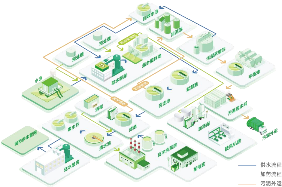
图 1：供水处理工艺流程介绍图示
