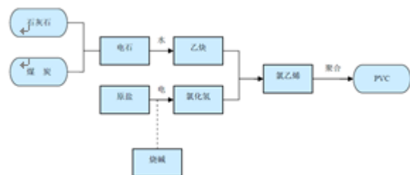
图 7：公司电石法 PVC 工艺流程
